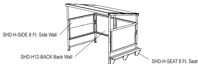
SHD-H12 136 W x 96 L x 113" H
